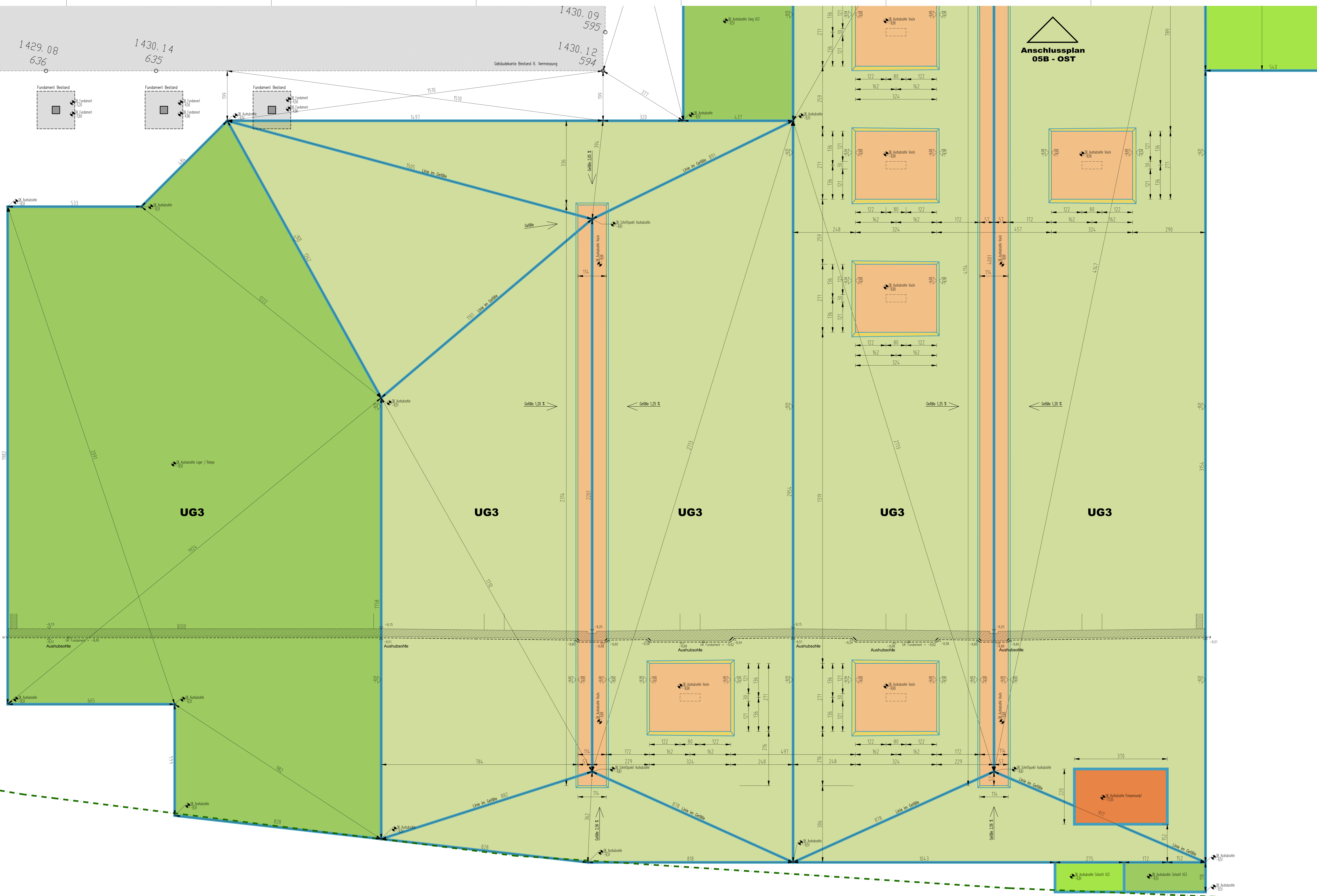
GRUNDRISS AUSHUBSOHLE
